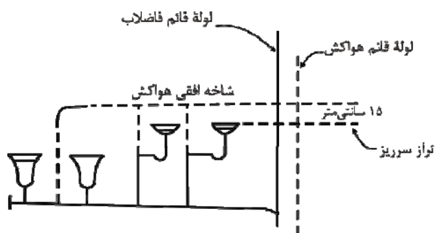
شکل ۵-۱۶-۲-۵ "پ" (۲) - اتصال هواکش به شاخه افقی لوله فاضلاب
