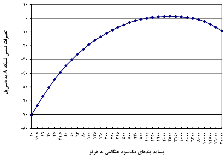
شکل ۱۸-۳-۶: نمودار تغییرات نسبی شبکه وزنی A در بسامدهای مختلف
