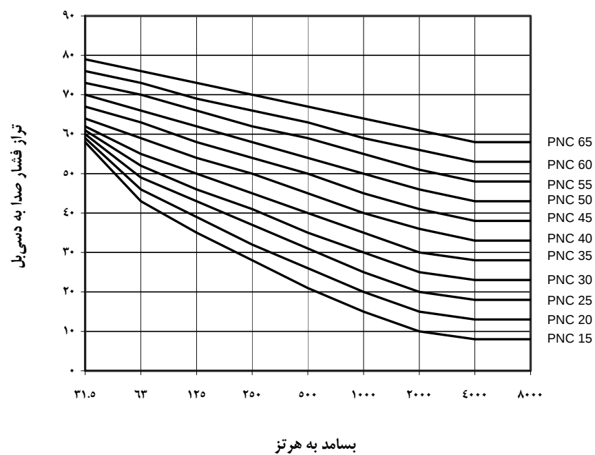
شکل ۱۸-۳-۵: نمودارهای پرسنج ترجیحی نوفه PNC
