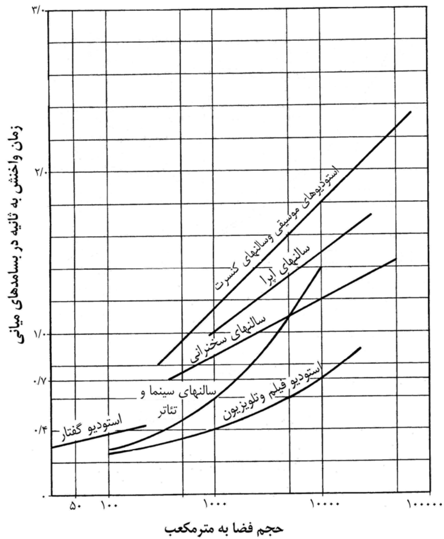
شکل ۲-۱۸-۱: نمودار زمان واخشن بهینه در فضاهای مختلف
