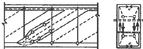
پ- عضو فشاری قطری در جان فارابی خاموت
