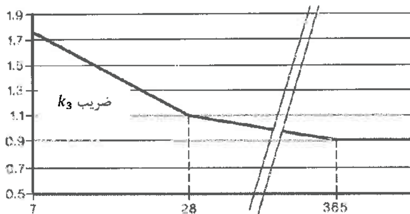
شکل ۹-۴-۱ ضریب k_3
