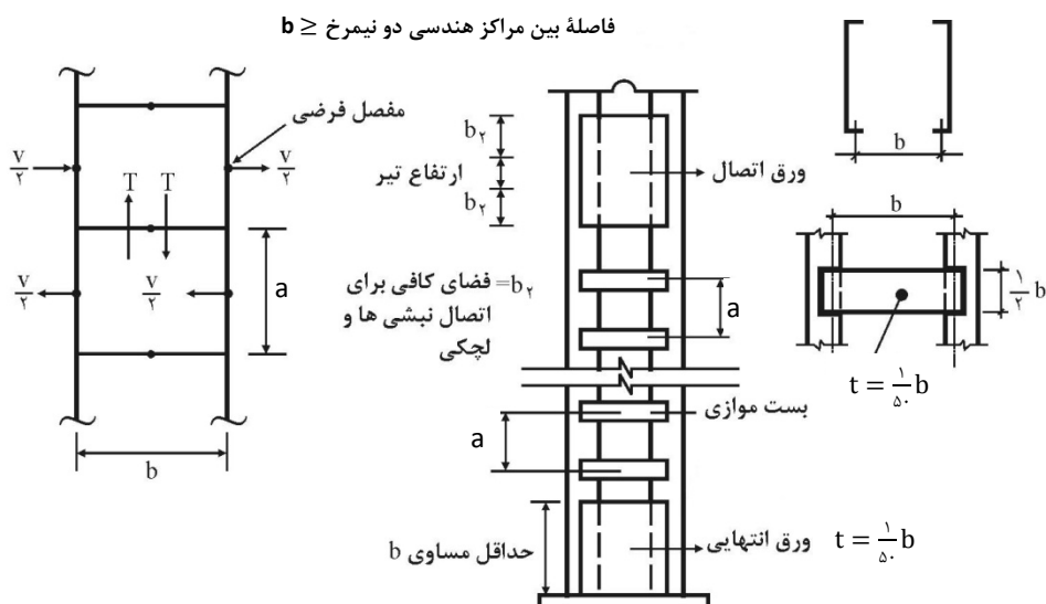
شکل ۱۰-۲-۴-۴ عضو فشاری ساخته شده با بست‌های موازی
