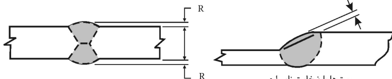
ورق ها با ضخامت مساوی
