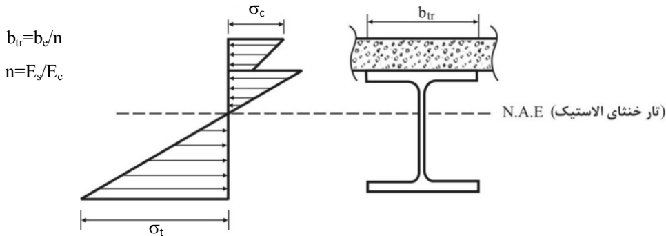
شکل ۳-۸-۱۰ توزیع الاستیک تنش در مقطع مختلط تبدیل یافته
