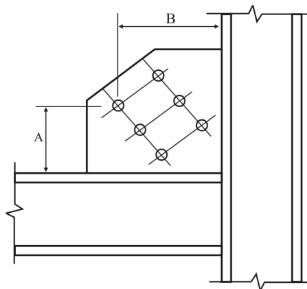
شکل ۱۰-۴-۱۴ رواداری مختصات سوراخ پیچ‌ها
