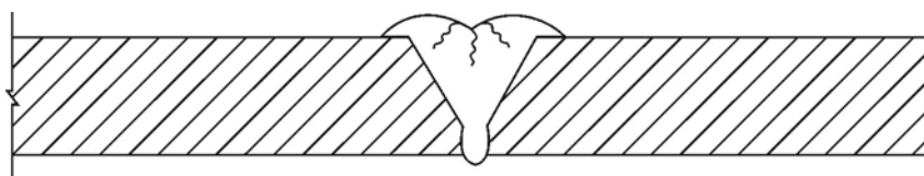
شکل ۱۷-۵-۶-۳-ب ترک های ستاره ای در سطح جوش.
