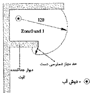
(۴) دید از بالا با موقعیت نصب دوش و دیوار جداکننده با حداقل شمع حد دسترسی از اطراف دیوار جداکننده
