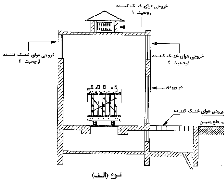
شکل ۵-۱۳-۳-۲: (نوع الف) - طرحواره مقطع قائم اتاق ترانسفورماتور خشک با تهویه طبیعی و هم سطح زمین
