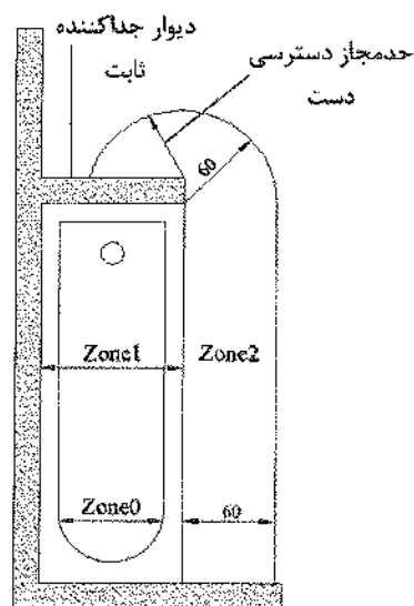
(۳) دید از بالا با دیوار جداکننده ثابت و خدمت‌جاز دسترسی
