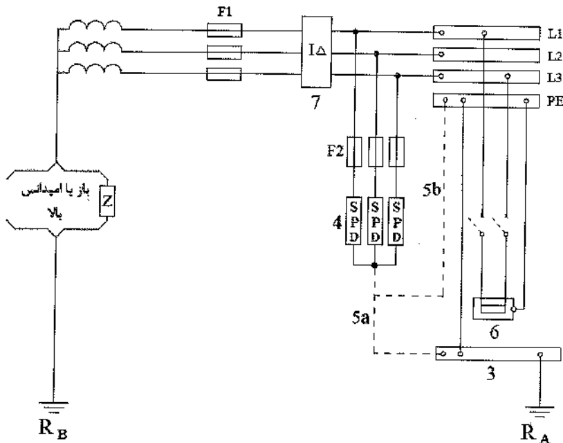
شکل ۴-۱۳-۱-۱۶-۴: طرحواره نصب برقگیر حفاظتی در شبکه توزیع سیستم نیروی IT
