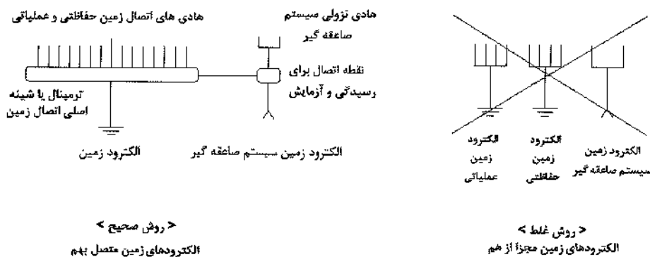
شکل پ ۱-۲-۸-۳ طرحواره نحوه اتصال الکترودهای زمین حفاظتی، عملیاتی و صاعقه‌گیر
