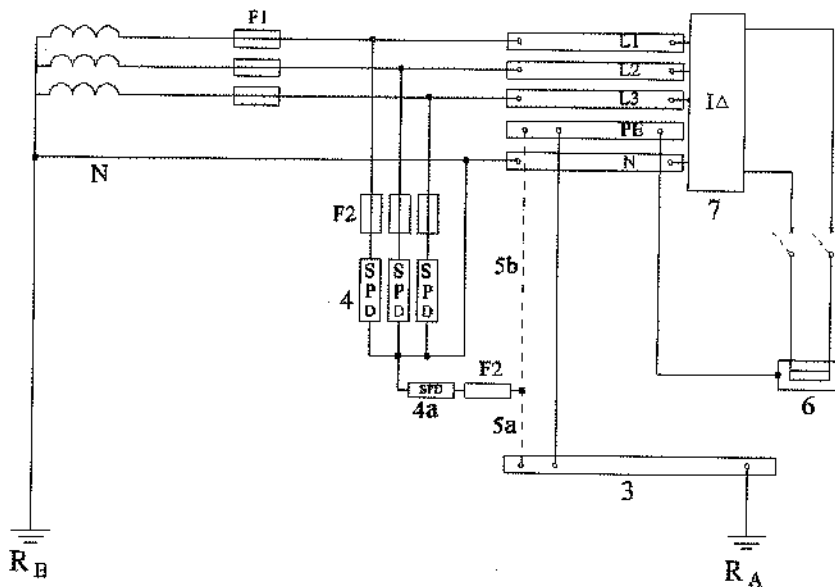
شکل ۳-۱۳-۱-۱۶-۴: طرحواره نصب برقگیر حفاظتی در شبکه توزیع سیستم نیروی TT با قرارگیری برقگیر حفاظتی قبل از کلید حفاظتی جریان باقی‌مانده (RCD)
